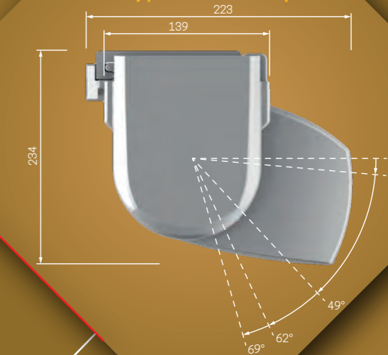
Bočný pohľad, rozmery a možný maximálne nastaviteľný sklon markízy pri montáži na strop
